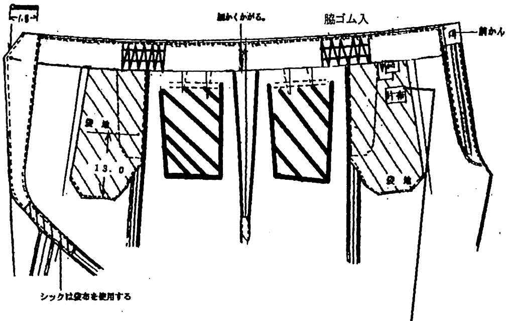
腰部裏図
