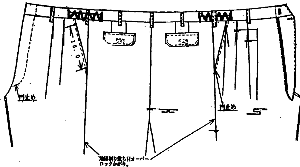
腰部裏図
